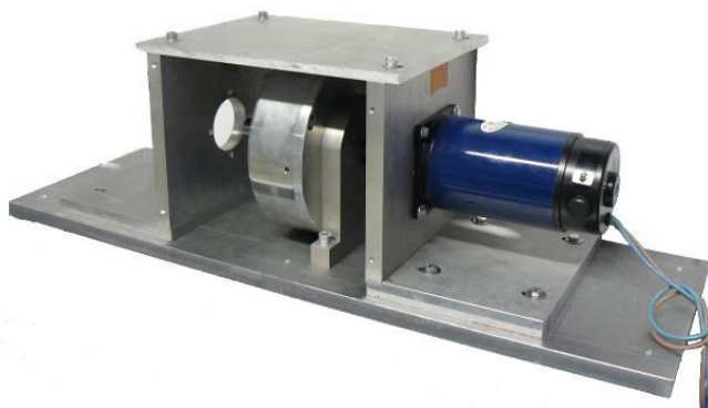
Banc d'essais couple moteur
